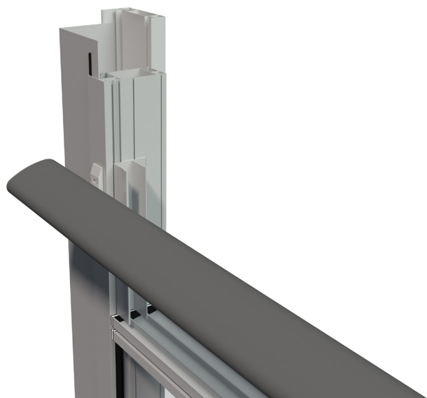
Twin Air med handledare. Tvärsnitt av hörnstolpe.
