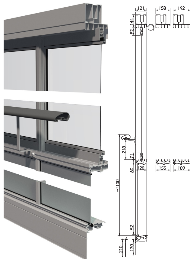
Twin Air. Tvärsnitt och ritning från sidan.
